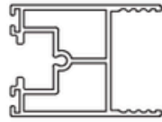
Baza Plinth
