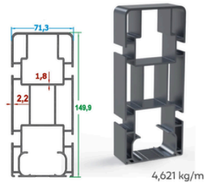
70'lık Eko Ray Profili | 70 Eco Rail Profile
