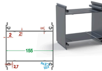
Dikme Profili Strut Profile
