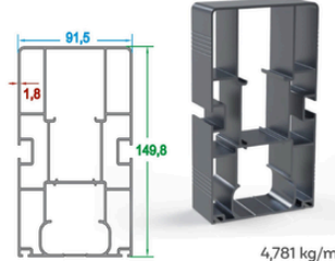
90'lık Orta Ray Profili 90 Medium Rail Profile
