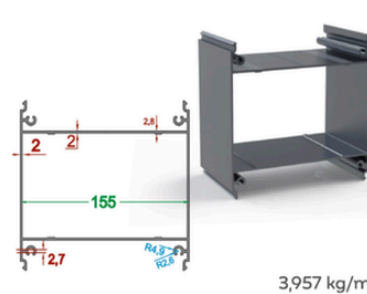
Dikme Profili Strut Profile
