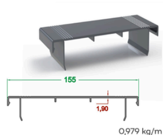
Dikme Kapak Profili Strut Cover Profile
