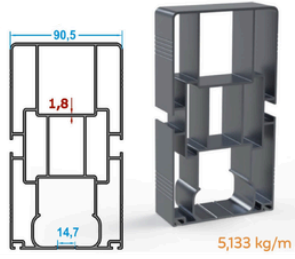
90'lık Eko Ray Profili | 90 Eco Rail Profile
